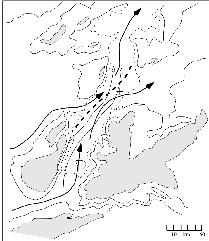
Abbildung 5.34: Schema der Mechanismen zur Erklärung der Unwetterzone der mittleren Oberrheinregion. Vgl. Abb. 5.23.
